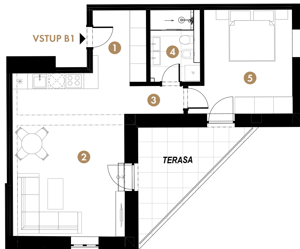
Pôdorys apartmánu
